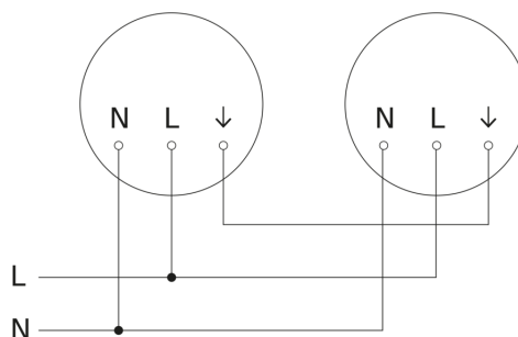
aansluitschema master/master
